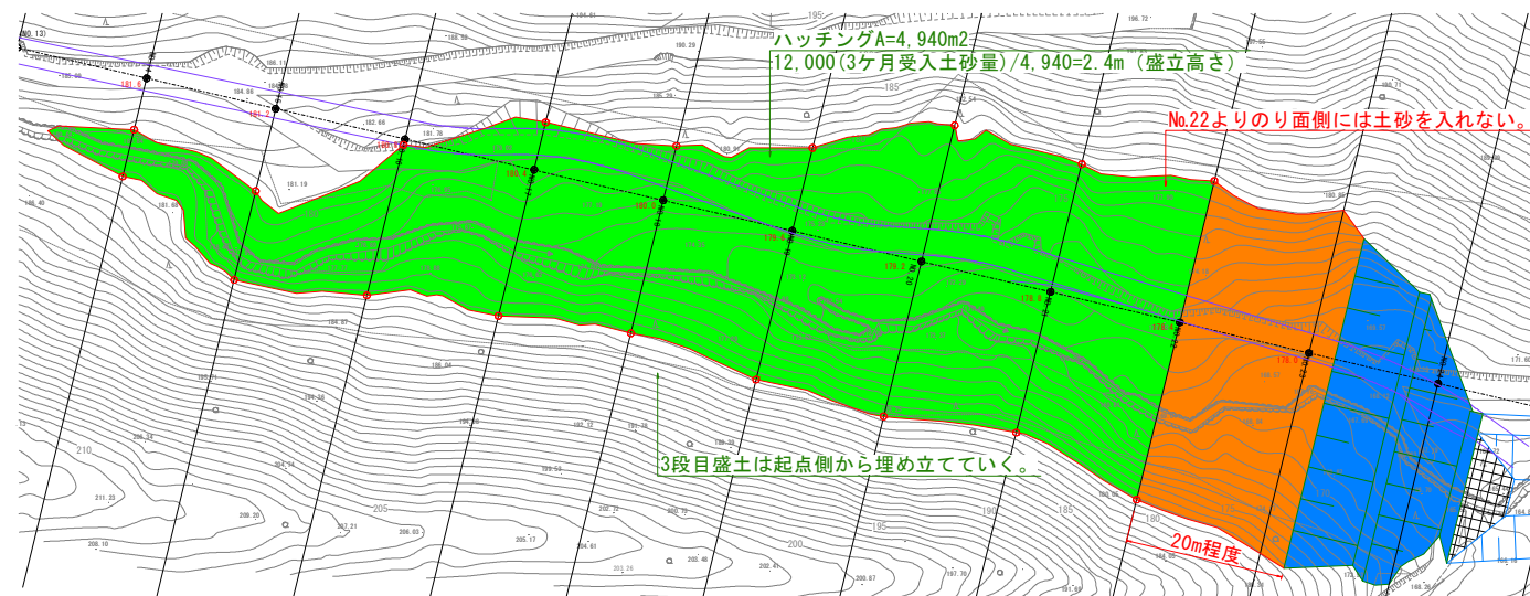
一次盛土完了時の平面図
