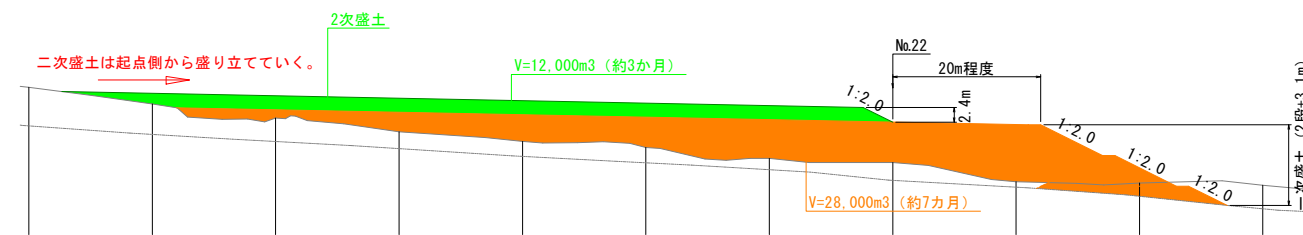
二次盛土の縦断図 (3 カ月)
