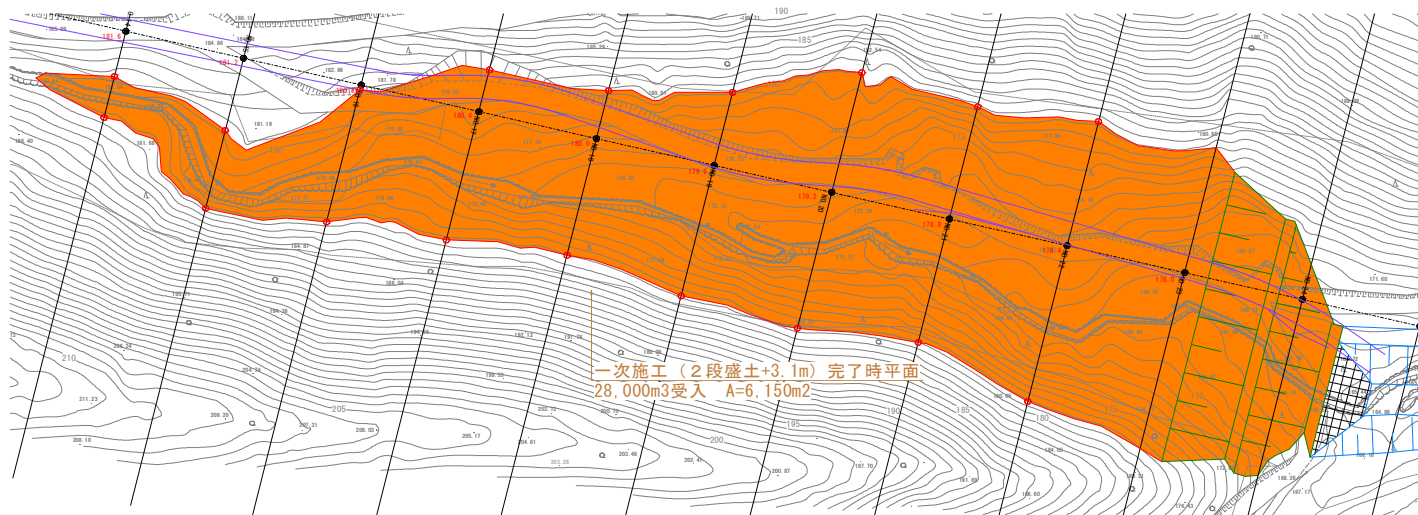
一次盛土完了時の平面図
