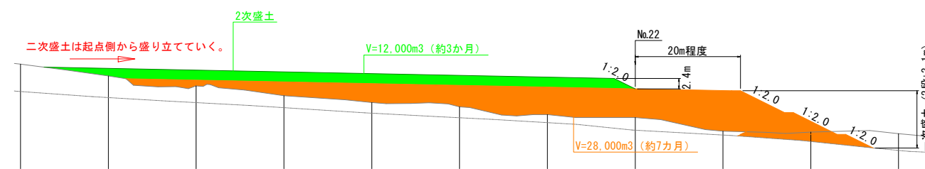
二次盛土の縦断図 (3 カ月)
