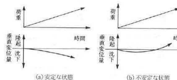
解図7-10 盛土のり面周辺地盤の鉛直変位の変化と基礎地盤の安定性の関係
