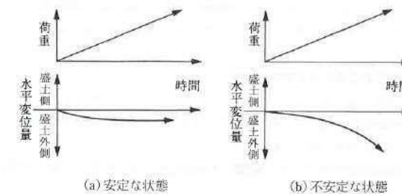
解図7-9 盛土のり面周辺地盤の水平変位の変化と基礎地盤の安定性の関係
