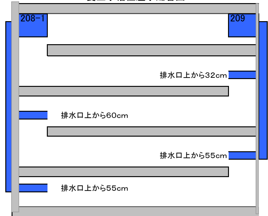
養生水槽恒温水配管図
