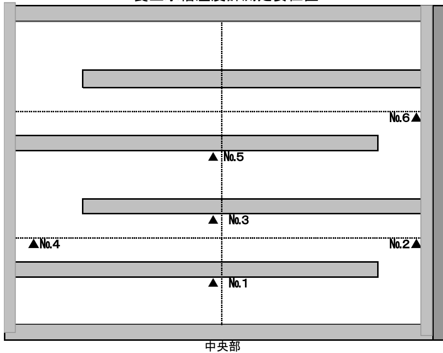
養生水槽温度計測定委位置
