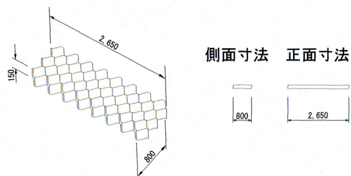
ジオセル工法 (R3) 形状図
